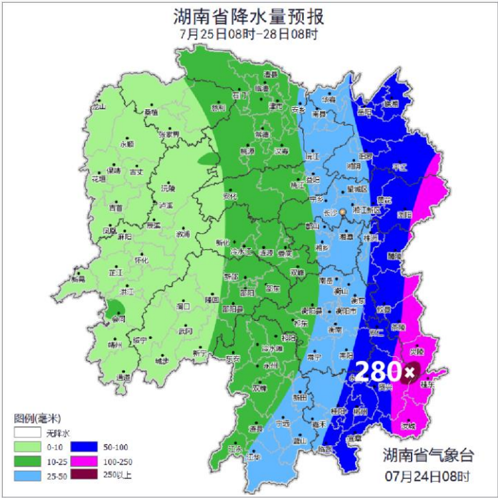
附图2 湖南省25日08时至28日08时累计降雨量预报图
