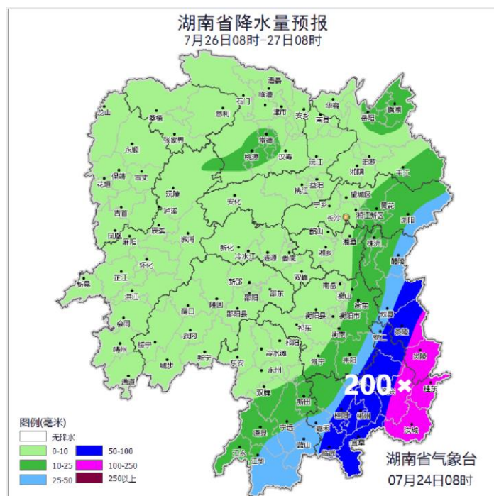
附图3 湖南省26日08时至27日08时降雨量预报图
