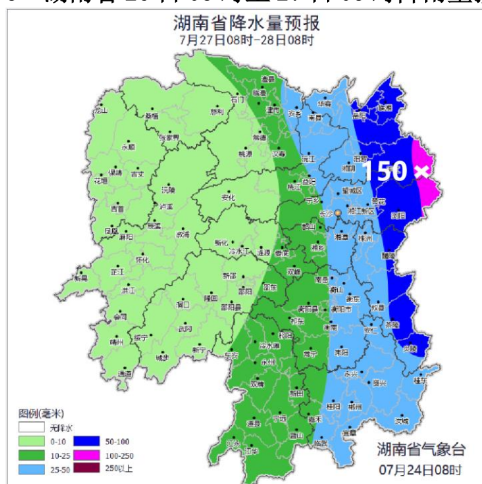
附图4 湖南省27日08时至28日08时降雨量预报图
