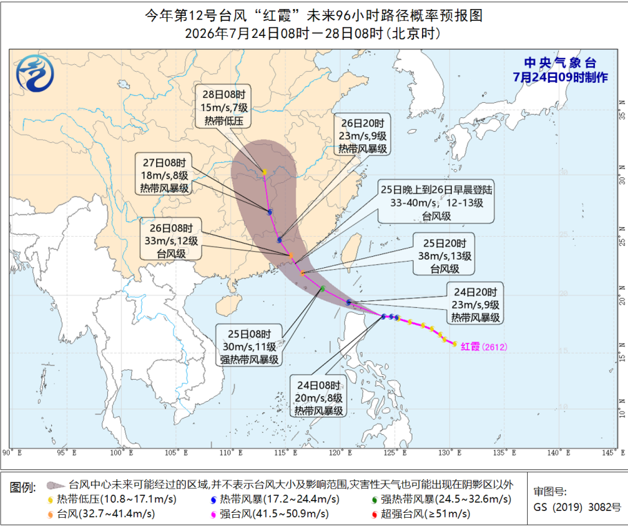
附图1 2026年第12号台风“红霞”未来96小时路径概率预报图
